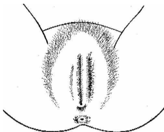
Zeichnung 2: Infibulation
