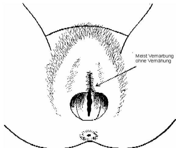
Zeichnung 1: Exzision
